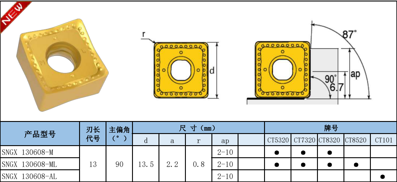
SNGX 刀片
