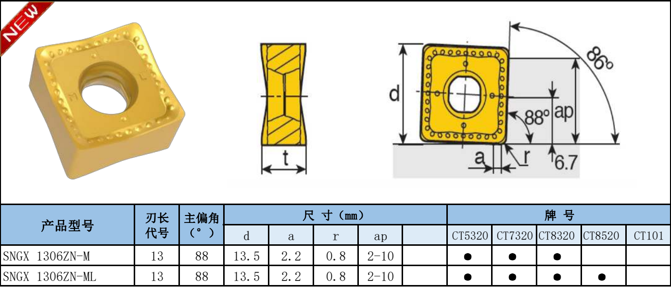
SNGX 刀片
