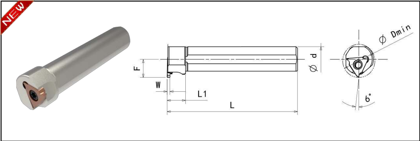
◎图示为右刀杆
