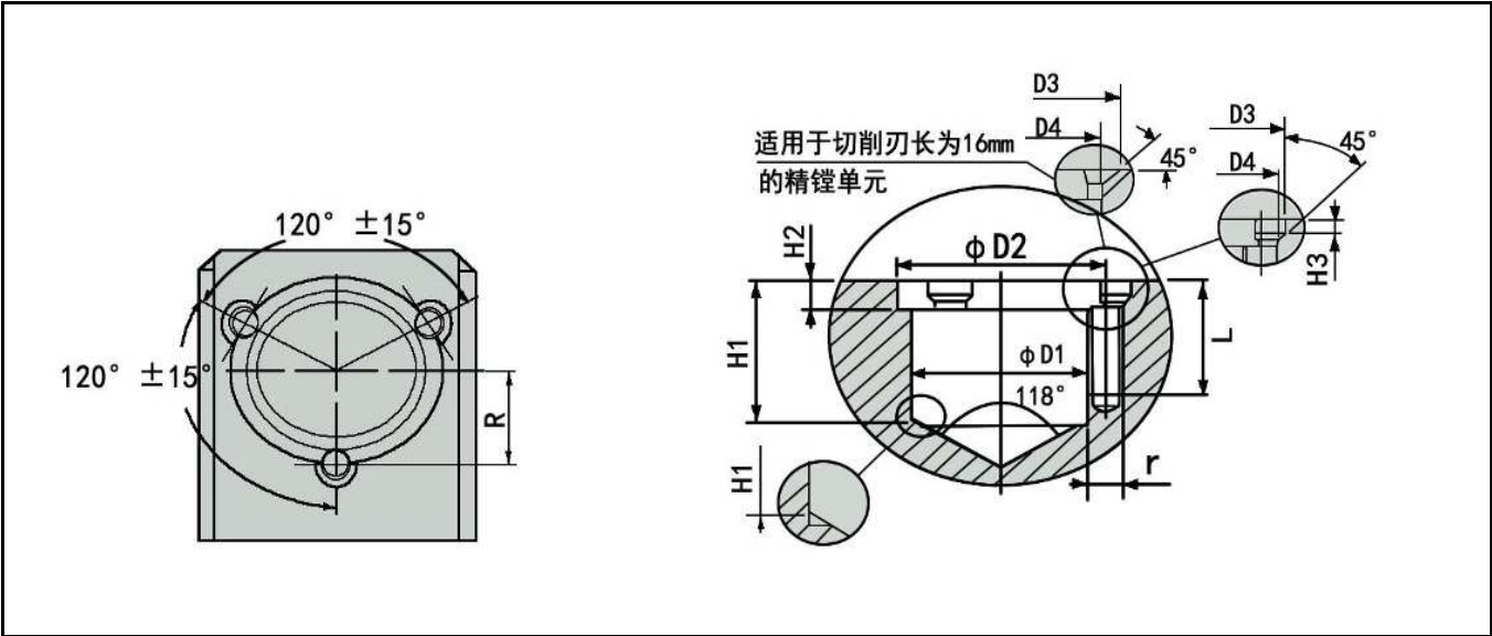
R/LCR微调精镗单元安装尺寸
